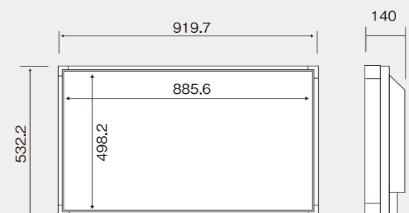
■ 40型マルチシンク液晶ディスプレイ(外形図) (単位:mm)
