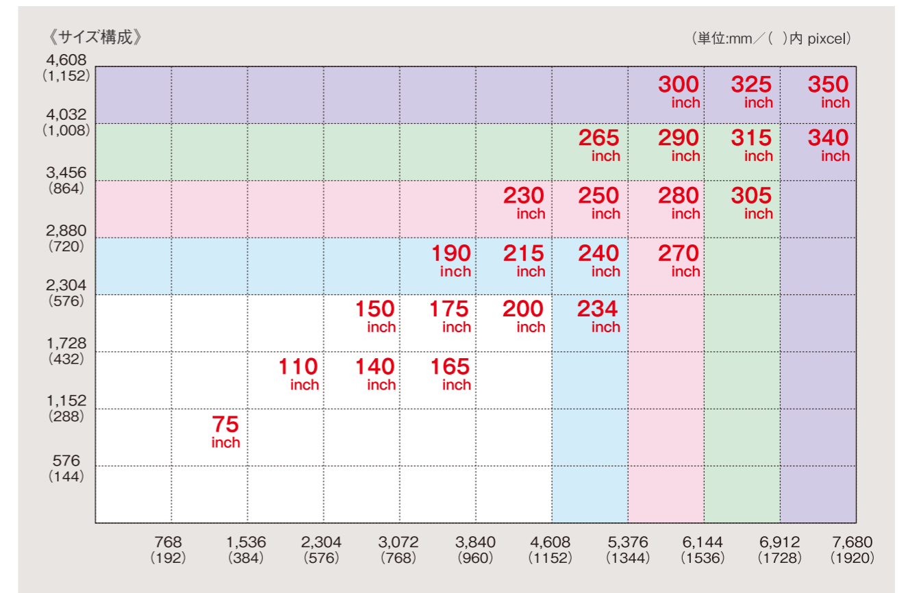
▲ ブラックフェイス/リアル4mmピッチ
